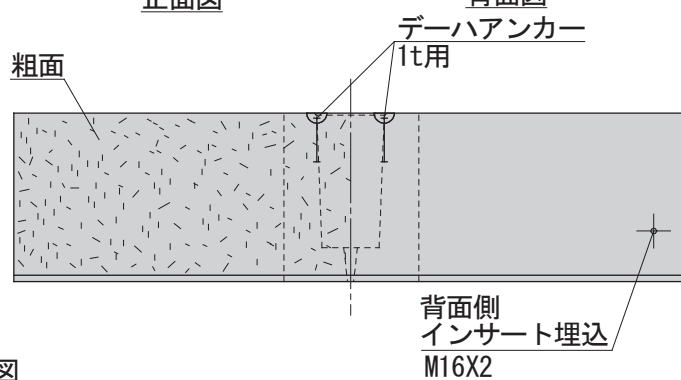
正面図
