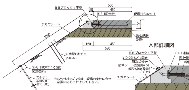
■BBシート工法 平型【路肩部 W=500】(100m当たり)
