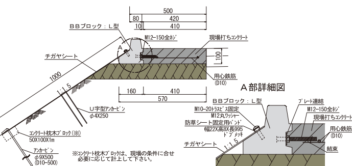
■BBブロック：L型
