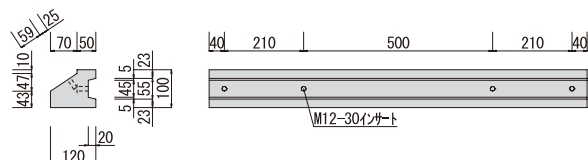
■BBブロック：平型
