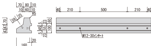
■BBブロック：L型
