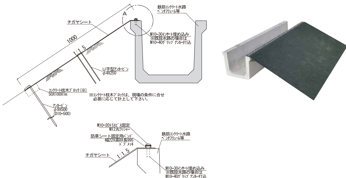
参考断面図および参考歩掛表
